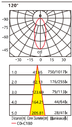
Q09-86 Claro REGLETA T8 120CM 20W
